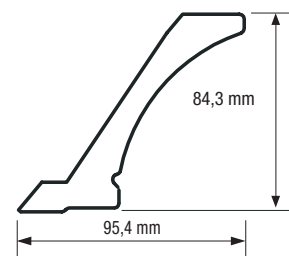
WP22 Moulure de tête contemporaine / Contemporary crown moulding Longueur / Length : 9 pi / ft
