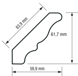
5027 Ogee régulier / Regular Ogee Longueur / Length : 9 pi / ft
