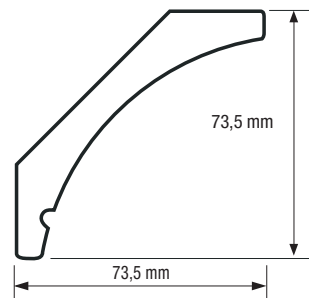
4766 Ogee concave / Concave Ogee Longueur / Length : 9 pi / ft
